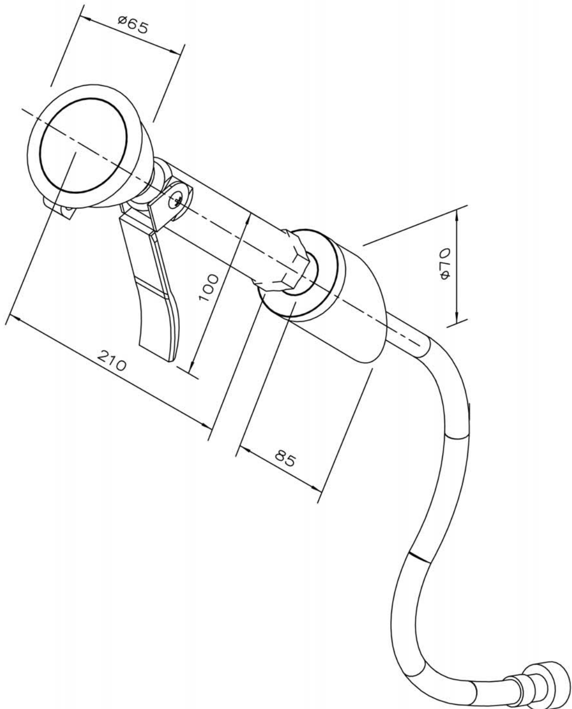
Wasseranschluss Augendusche Waterinlet eyewash G 1/2" IG female
